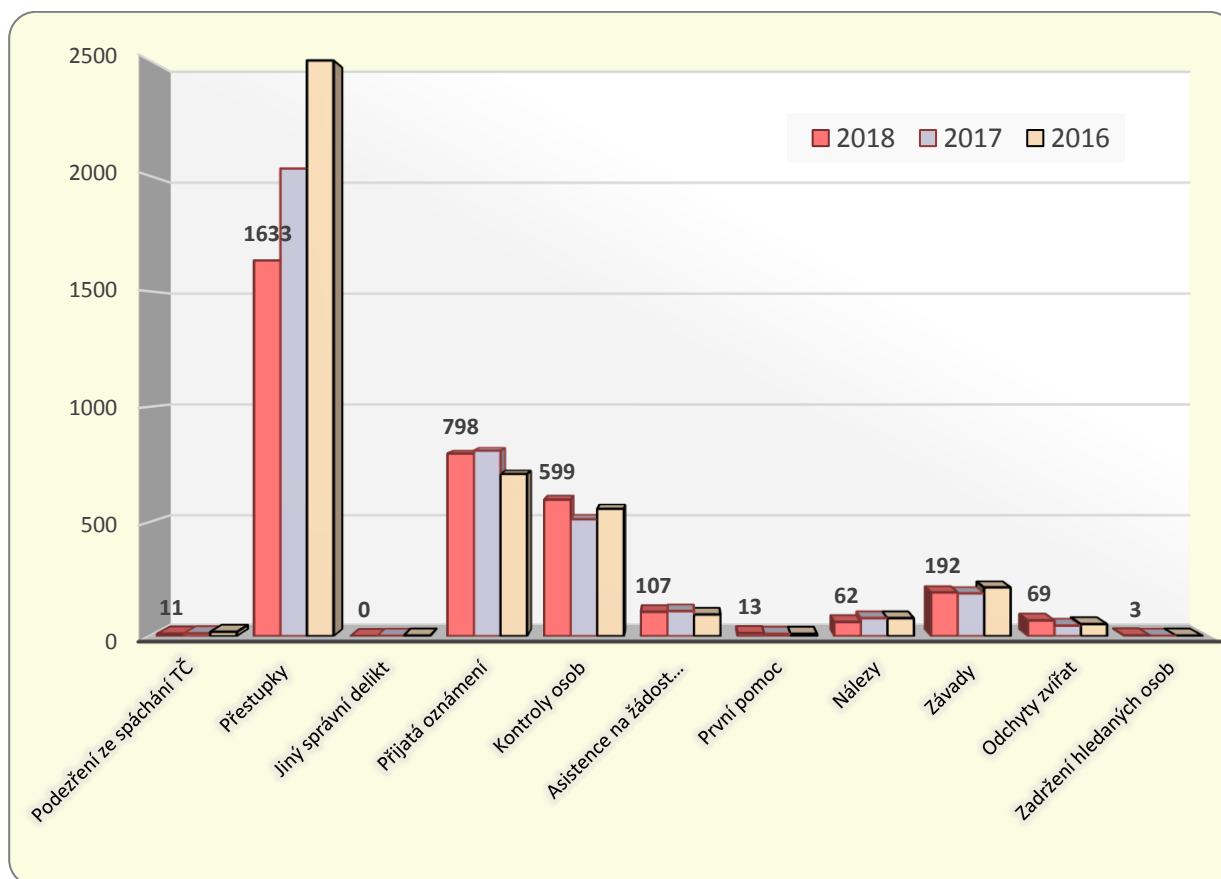
Graf 1: Rozložení evidovaných událostí - porovnání let 2016, 2017 a 2018 (Bolom, 2019)
