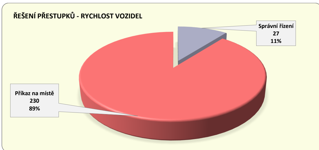
Graf 4: Řešení přestupků - rychlost vozidel 2018 (Bolom, 2019)
